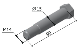
Болт Р33.11.04.104 М = 0,162 кг
