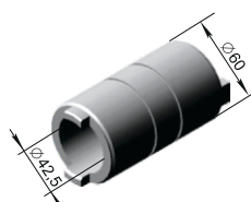
Втулка СЗР.00.811 (на сеялку СЗС-2) М = 1,18 кг
