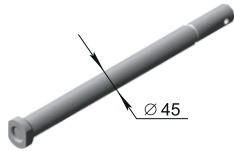
Ось батареи БДО 01.625/ БДО 16.626 L = 1700, M = 21,2 кг L = 1920, M = 23,96 кг
