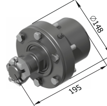
Ступица Р33 24.07.500 СБ M = 9,5 кг
