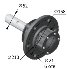
Ступица колеса ПНЛ.РЗЗ.16.100 М = 22,56 кг
