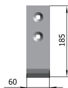
Долото Р33 КША.25.050 М = 0,86 кг
