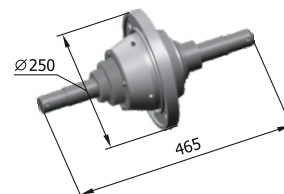
Ступица с осью Р33.39.05.100-01СБ М = 23,6 кг
