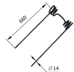
Зуб пружинный к бороне БЗГ (14мм) 47.664.04.002 М = 4 кг
