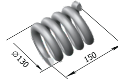
Пружина Р33.22.04.002-01 M = 5,5 кг
