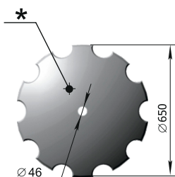
Диск БДТ Р33.428.001 лист-6 (на бороны) М = 15,3 кг
