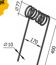
Зуб пружинный к бороне БЗГ 47.565.04.001 М = 1,2 кг
