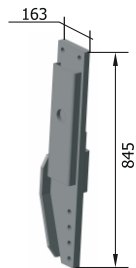
Стойка (литьё) РЗЗ.89.01.200 М = 35,8 кг
