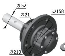
Ступица Р33.16.100 М = 22,56 кг
