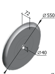
Каток СЗЮ.00.160 М = 13 кг
