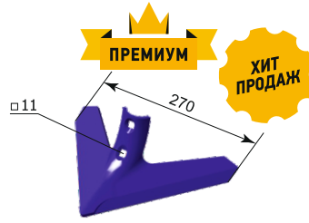
Лапа «Омычка» (270 мм) СКС.01.08.080-02 Алмаз (65г) М = 1,1 кг
