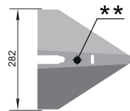
Лапа СКП.03401 (стелс) М = 2,1 кг
