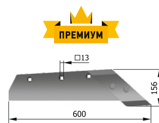
Лемех с доломом правый Р33.11.31-400 М = 6,9 кг
