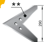
Лапа С4 (290 мм) РЗЗ.АУП.18.02.020Г М = 1,1 кг
