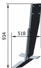
Рабочий орган Р33.ПСК.ЧГ.300 М = 44,6 кг
