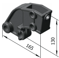
Держатель КПЦ 00.207 М = 1,8 кг
