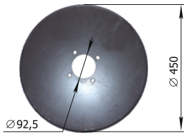
Диск сошника сеялки «Bourgault» 47.771.001 М = 5,46 кг
