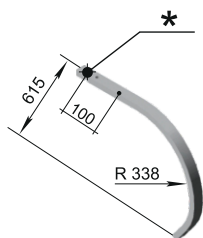
Стойка Р33.043.13.401 М = 13,15 кг
