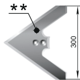
Лапа сеялочная (300 мм) СКС.01.08.080-01 М = 1,38 кг
