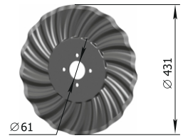
Турбодиск зубчатый «Томь» 47.1221.001 М = 4,6 кг
