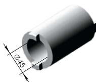
Втулка СЗР.00.809 (на сеялку СЗС-2) М = 1,2 кг
