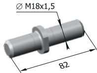
Шпилька Н130.05.607 M = 0,18 кг
