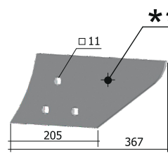
Отвал предплужника РЗЗ.П. 2-В М = 1,8 кг
