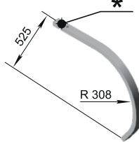
Стойка РЗЗ,043,13,401-02/01 М = 12 кг
