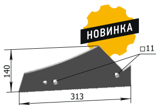
Грудь отвала ПЛП.01.004 М = 1,5 кг
