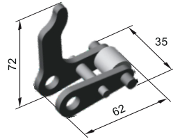
Защелка СЗГ 00.600СБ М = 0,15 кг
