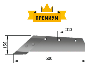
Лемех с доломом левый Р33.11.51.400 М = 6,9 кг
