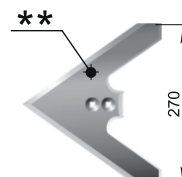
Лапа (270 мм) Р33.00.130 М = 1,15 кг
