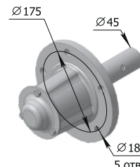
Ступица колеса ПЛЕ РЗЗ.06.200-Б М = 13,66 кг
