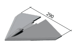
Лапа сошника РЗЗ.АУП.18.02.020Г М = 1,84 кг
