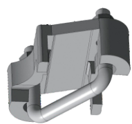
Державка предплужника в сборе Р33.215.00.000-01 М = 4,4 кг
