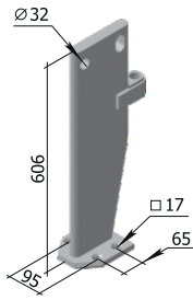
Стойка КША.25.010 М = 26,6 кг
