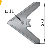
Лапа сеялочная «Омычка» (270 мм) СКС.01.08.080-02 М = 1,1 кг
