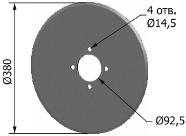
Диск сошника сеялки «Semeato» 47.1074.001-01 М = 4,29 кг
