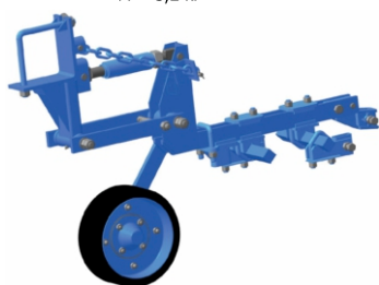
Секция КРН Р33.КРН.71.00.000 М = 51 кг
