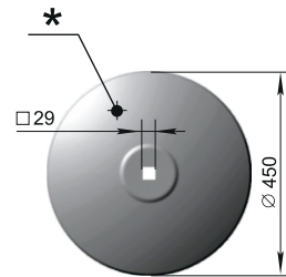
Диск ЛДГ С-1-1-450-5-29 Р33 407.001 М = 6,25 кг
