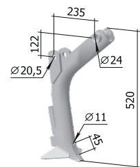
Стойка СКП 01.08.060 «Омичка» М = 5,5 кг
