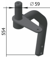
Стойка для дискаторов с развернутым диском Р33.25.20.100-01 M = 18,4 кг
