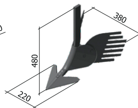
Корпус очучника 2Н.082.04.000-18 М = 8,54
