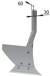
Предплужник без державки РЗЗ.02.010 М = 17,8 кг
