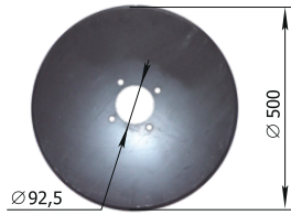
Диск сошника сеялки «Bourgault» 47.771.001-1 М = 7 кг
