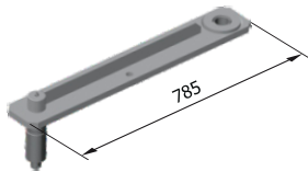
Рычаг 4x4.07.04.000-02 M = 21,7 кг
