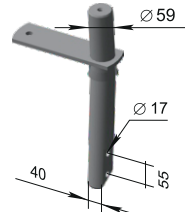
Стойка Р33.47.01.100 M = 11,1 кг
