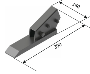
Наральник Р33.ПЧН-2,7 М = 9,2 кг
