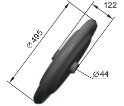
Каток СЗСА 01.23.001 М = 8,6 кг
