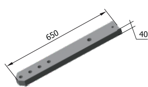
Стойка Р33.11.51.006-02 М = 18,5 кг
