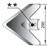
Лапа Salford (290 мм) РЗЗ.290604.00 М = 2,07 кг
