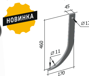
Стойка КСО Н.043.11.401-05 М = 2,67 кг
