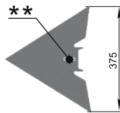
Лапа (375 мм) РЗЗ.ТЗ94.08.00 М = 2,94 кг
