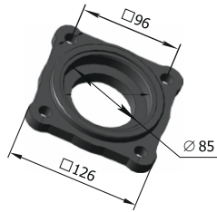
Крышка корпуса подшипника Р33.БДЛ-322 M = 1,09 кг
