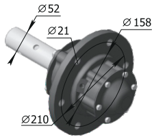
Ступица колеса ПНЛ.Р33.16.100 М = 22,56 кг
