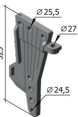
Стойка (литьё) РЗЗ.ПЛЕ 31.301 М = 17 кг
