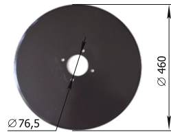
Диск сошника сеялки «John Deere 1895, 1890» 47.469.02.001 М = 5,8 кг
