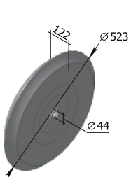
Каток СЗШ.00.370 М = 9 кг
