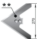
Лапа сеялочная (270 мм) СКС.01.08.080 М = 1,17 кг
