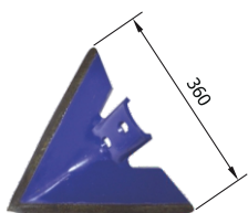
Лапа «Кузбасс» 47.917.001 М = 2,4 кг
