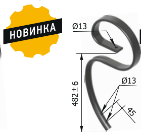
S-образная стойка 45x12 47.1202.02.02.002-02 М = 5,2 кг
